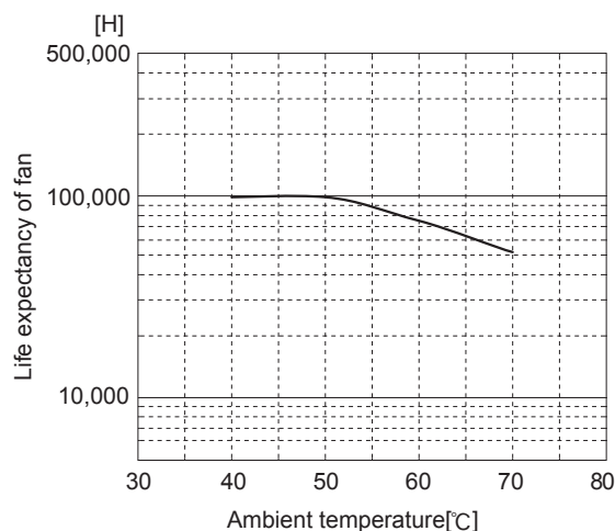
Fig.5.2 Life expectancy of fan (PDA600F)
