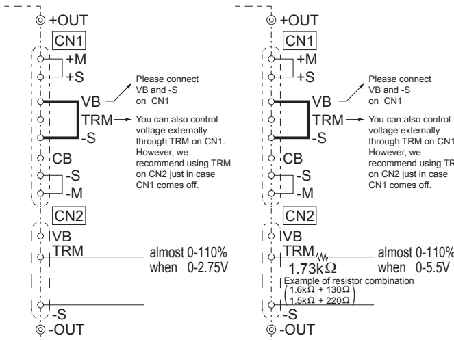
Fig.1.1 Wiring 1
