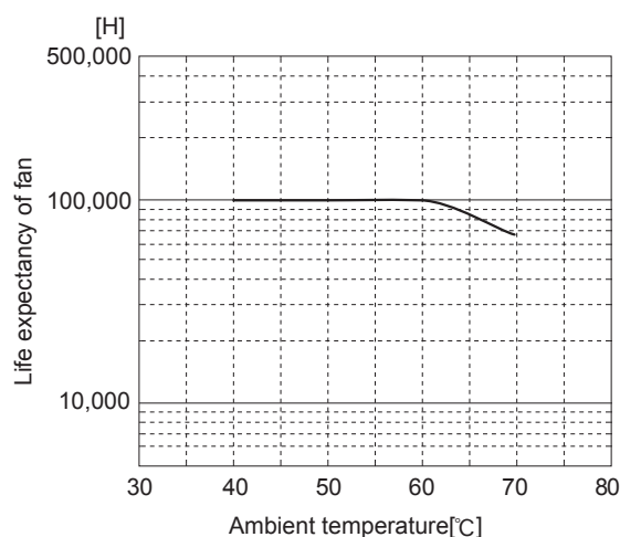
Fig.5.1 Life expectancy of fan (PDA300F)
