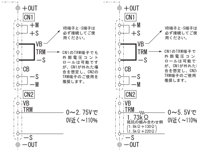
図 1.1 配線 1
