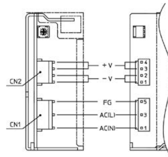
図 8.1 - J1 仕様の例 (PDA50F)
