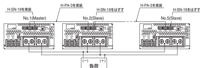
図3.3 並列運転時の接続（PDA600Fの例）
