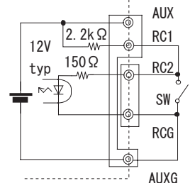
図 1.5 リモートコントロール回路接続例
