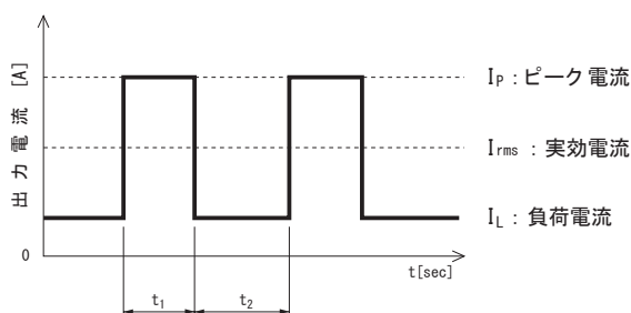
図2.1 ピーク電流
