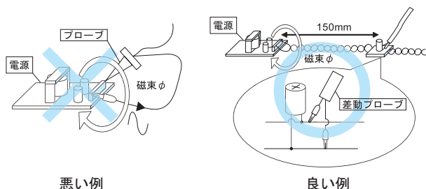
図 1.4 出力リップル・リップルノイズ測定例
