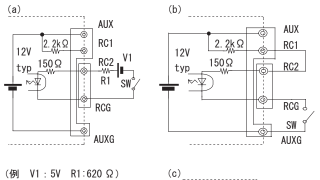
図 1.5 リモートコントロール回路接続例
