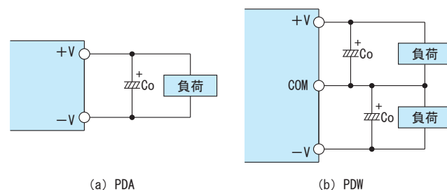
図7.2 出力側外付けコンデンサ接続方法
