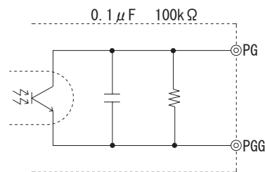
図 1.8 PG 信号の内部回路
