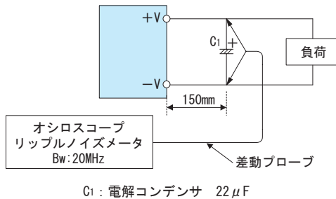
図 1.3 出力リップル・リップルノイズ測定方法
