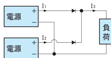
図3.2 冗長運転例
