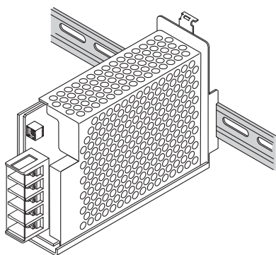
図 8.2 DIN レール取り付けイメージ図 (PDA50F)
