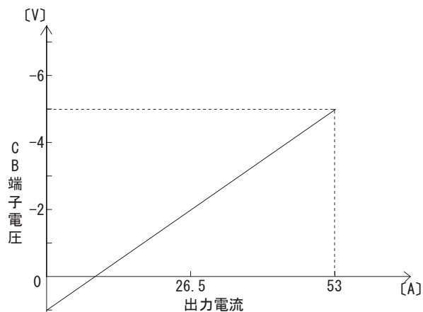
図 7.1 出力電流－CB 端子電圧 (例：PDA600F-12)
