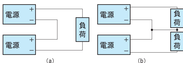
図3.1 直列運転時の接続例
